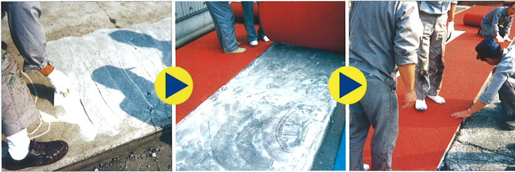
1. 路面に接着剤を塗布(くし目で) 2. その上にクッションマットを被せる 3. 乾燥すれば完成
